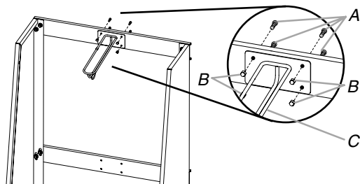
A. Tornillos Phillips (F3b) B. Tuercas ciegas hexagonales (F10) C. Divisor para la bolsa de golf
