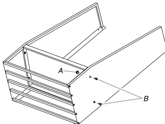
A. Tuercas de reborde de 5/16" (F2)
