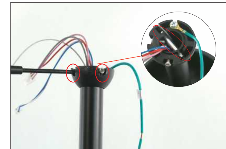
Paso 9 Aprieta el tornillo de la semiesfera.
