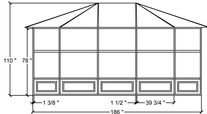
VUE DE CÔTÉ (LONGUEUR) SIDE VIEW (LENGTH)
