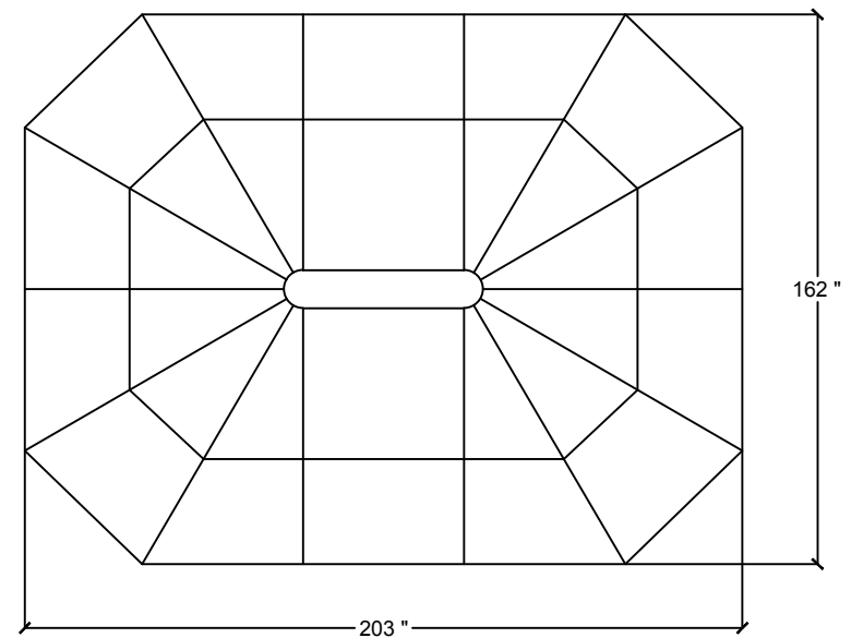
REBORD DU TOIT ROOF OVERHANG
