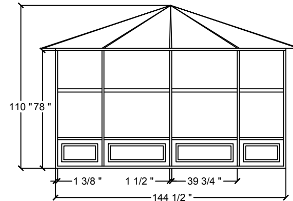
VUE DE CÔTÉ (LARGEUR) SIDE VIEW (WIDTH)
