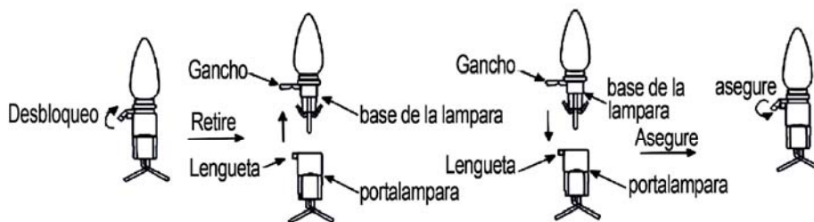
Fig.1 Desbloquee y retire la lámpara quemada
