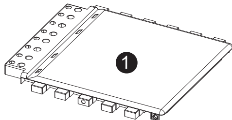
Seat Frame QTY:2
