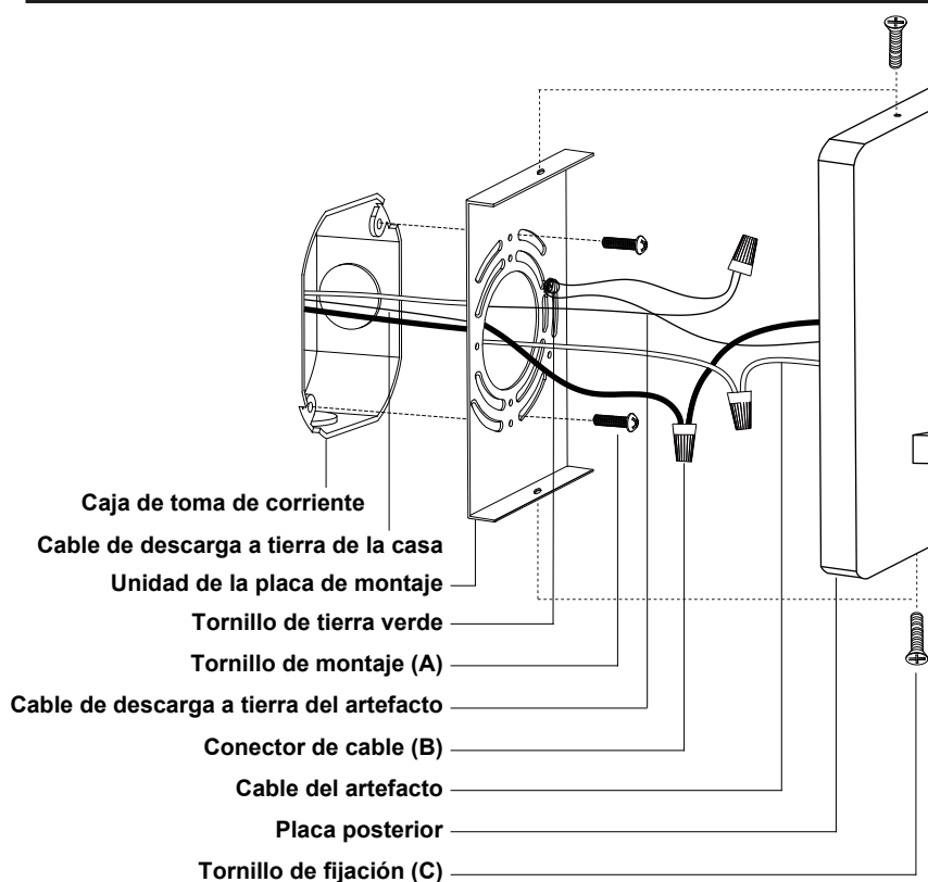
Tornillo de fijación (C) (se incluyen 2 adicionales)
