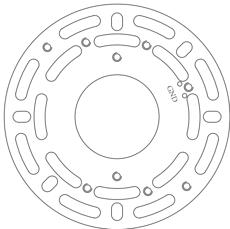
Placa de montaje redonda (no está a escala)
