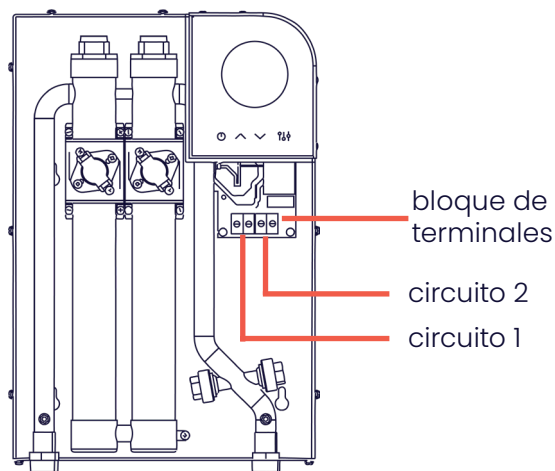
VISTA FRONTAL SIN CUBIERTA
