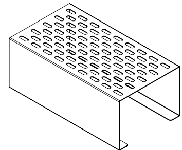
Figure 26 Étagère de congélation, modèle RF uniquement
