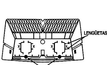
CARCARSA DELANTERA DEL FILTRO LAS UBICACIONES DE LOS FILTROS ESTÁN MARCADAS CON UNA X
