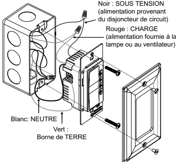
Fig. 3. Orientation de l'interrupteur, raccordement des fils et ensemble de boîtier mural
