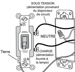
Fig. 1. Branchement typique d'un interrupteur unipolaire
