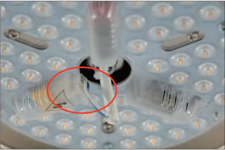
Paso 14 Conectar el cable de alimentación de la luz
