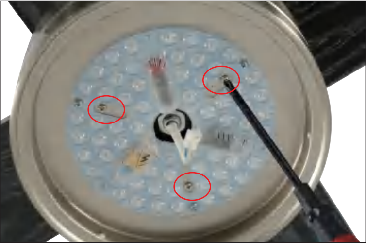
Paso 15 instale la placa de la luz.
