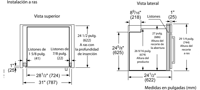
Instalación a ras
