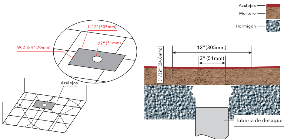
Diagrama de sección transversal del piso
