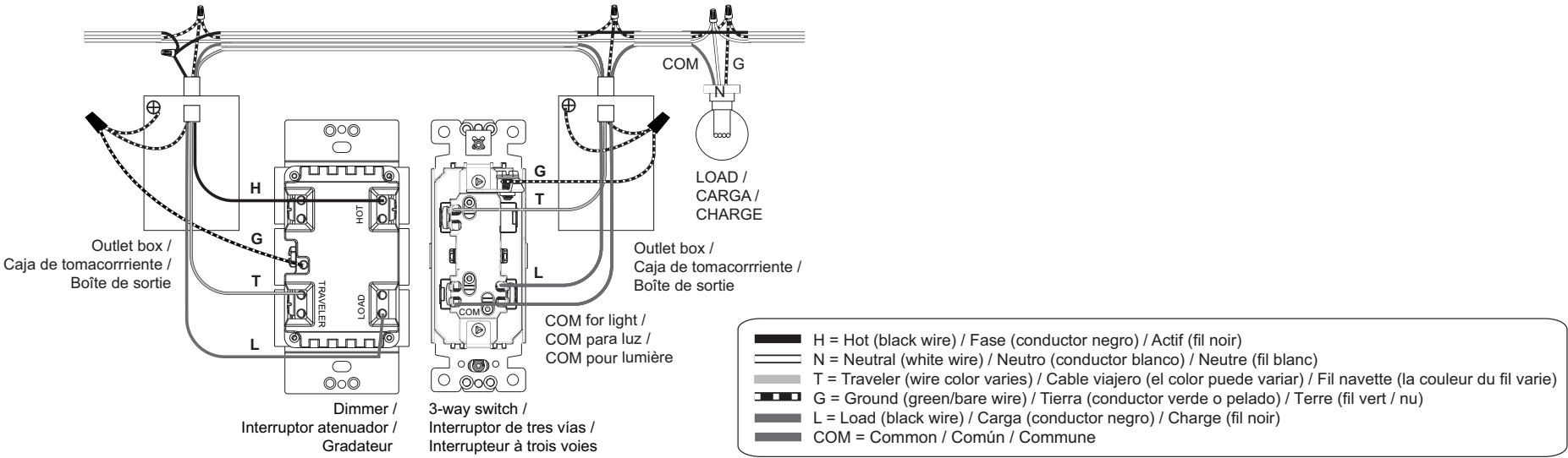
Figure / Figura / Figure 2 : 3-Way Wiring Diagram / Diagrama de cableado de tres vías / Schéma de câblage d'un interrupteur à 3 voies
