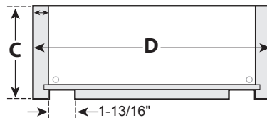
Drawer Front / Parte frontal de la gaveta
