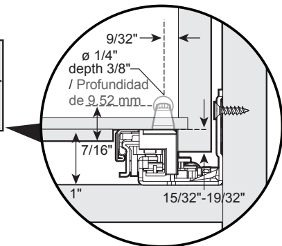
Drawer Front / Parte frontal de la gaveta
