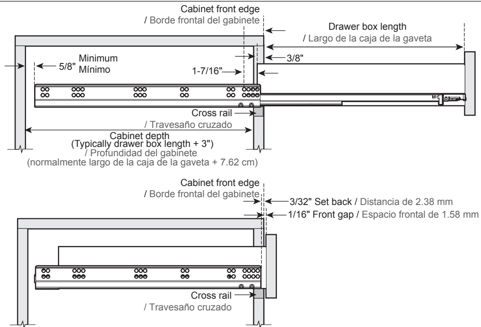
Cabinet Front / Parte frontal del gabinete
