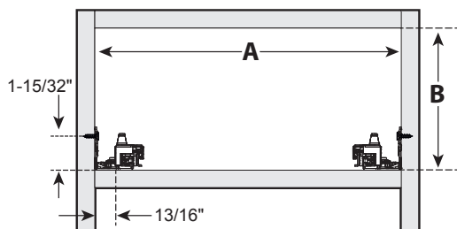
Cabinet Front / Parte frontal del gabinete
