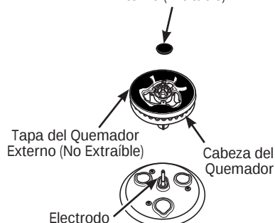
Quemador de Tres Anillos (en algunos modelos)
