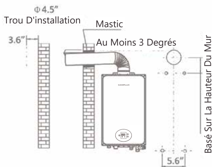
Installation Latérale
