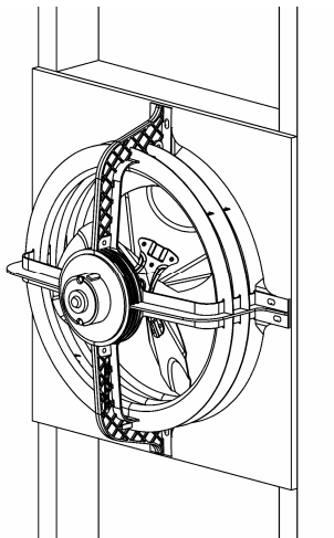
Illustration – 3 Installed Fan Assembly Ilustración – 3 Conjunto del ventilador instalado
