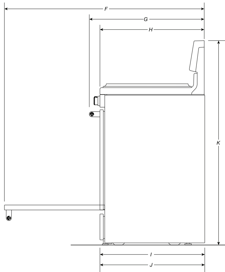
VUE LATÉRALE
