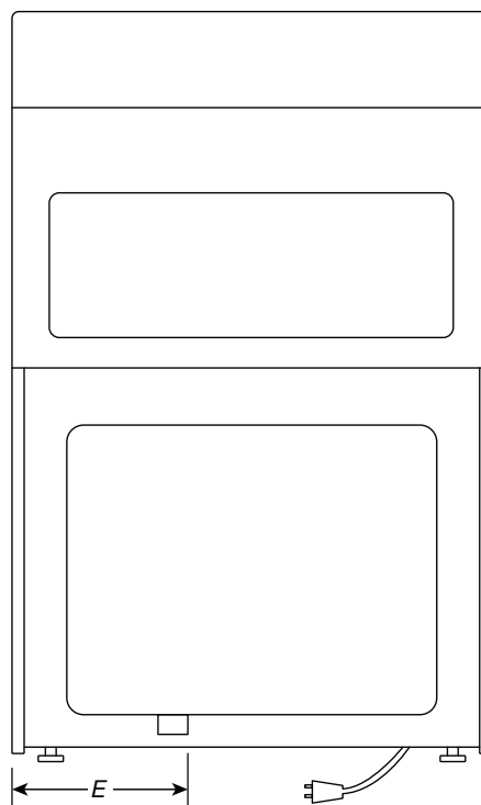
VISTA POSTERIOR
