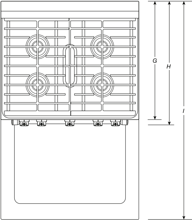
VISTA SUPERIOR
