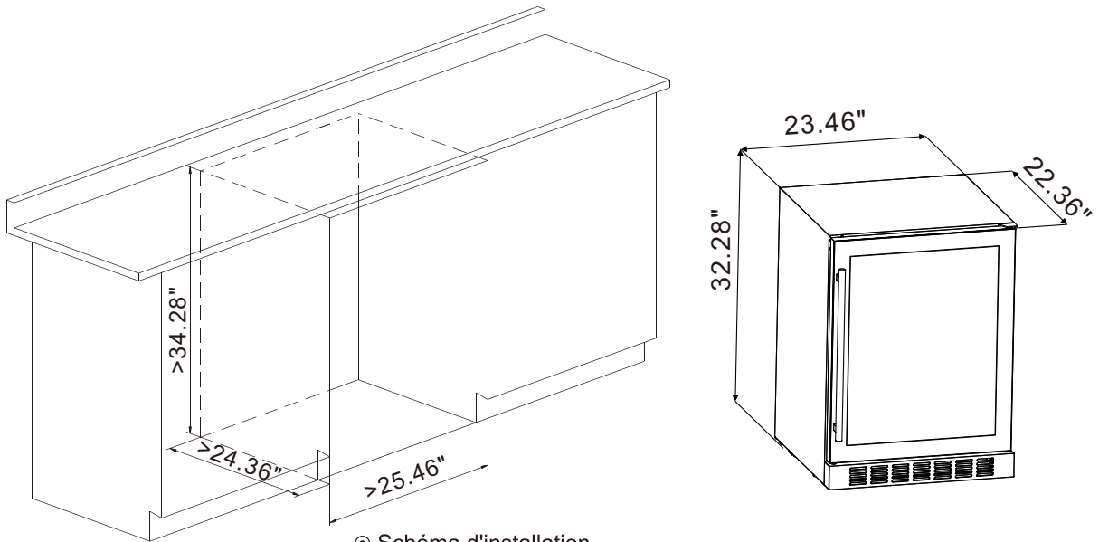
© Schéma d'installation
