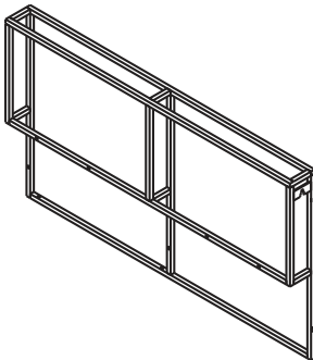
Left back frame (1 pc)
