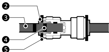
2 Collet 3 Tube 4 Ligne d'insertion 5 Attache
