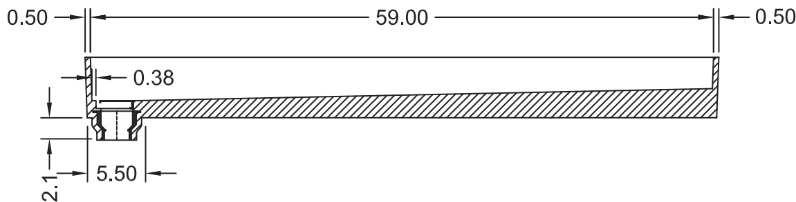
SECTION A-A
