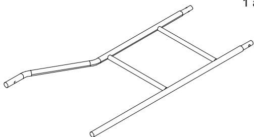
(C) 2 Legs (1 right and 1 left) 2 Soportes (1 derecho y 1 izquierdo) 2 montants (1 droit et 1 gauche)
