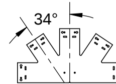
56619 8:12 Truss Base Fan (TBF-8-12)
