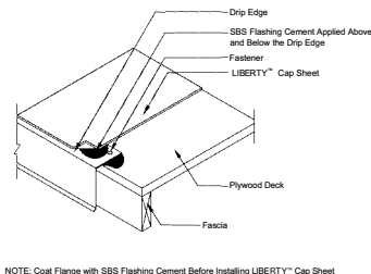
Edge Flashing
