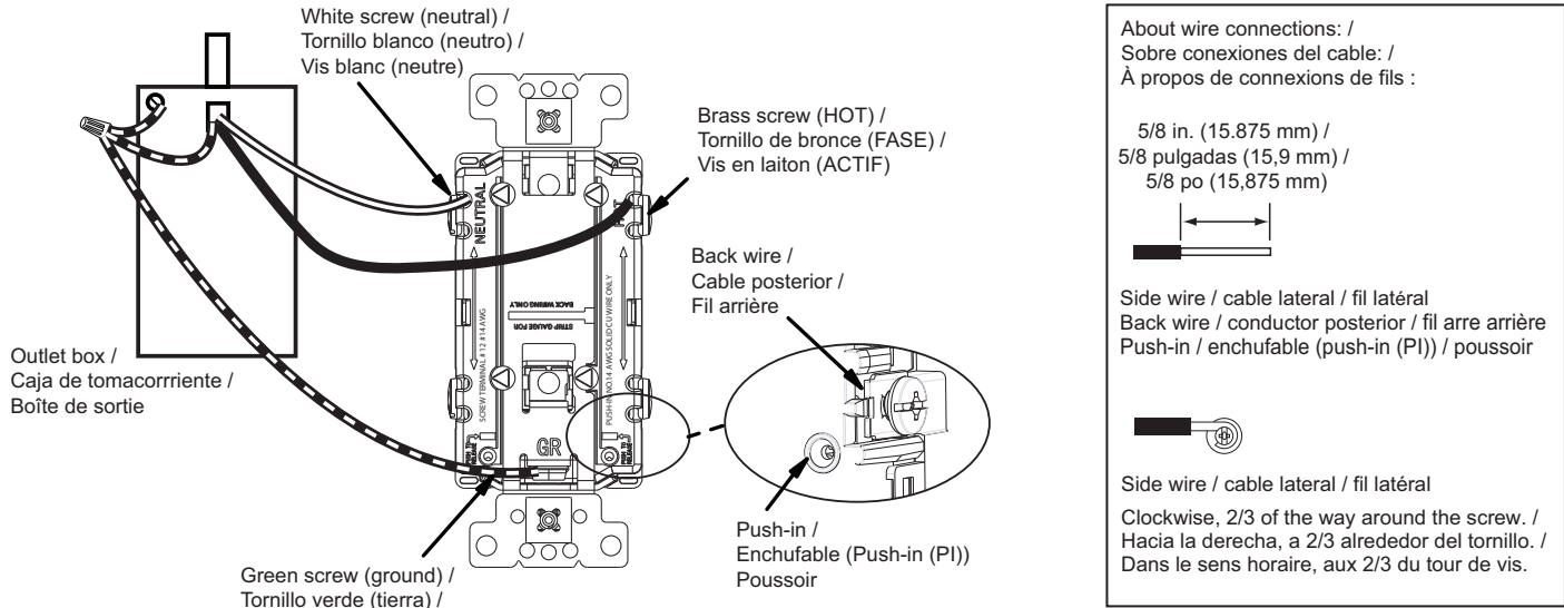
Figure / Figura / Figure 1 : Wiring Diagram / Diagrama de cableado / Schéma de câblage
