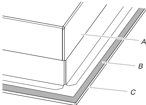
A. Base de la table de cuisson B. Bande de mousse de \frac{1}{4} " (0,64 cm) C. Table de cuisson
