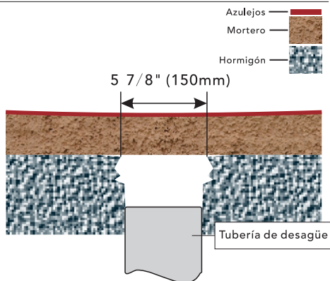
Diagrama de sección transversal del piso
