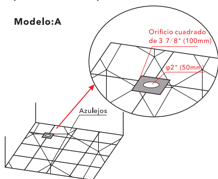
Piso del baño inclinado Vista desde arriba
