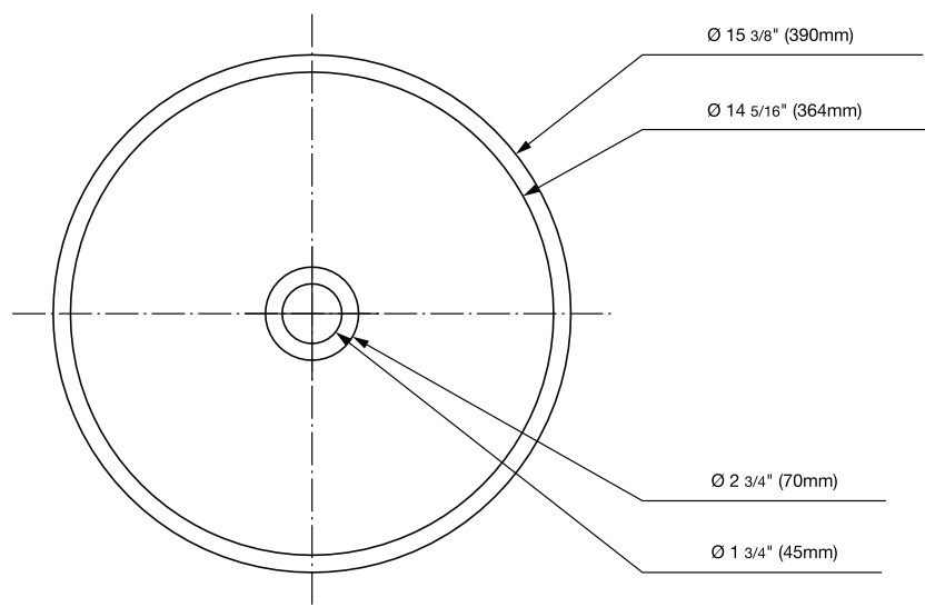
TOP VIEW / VISTA SUPERIOR / VUE DE HAUT
