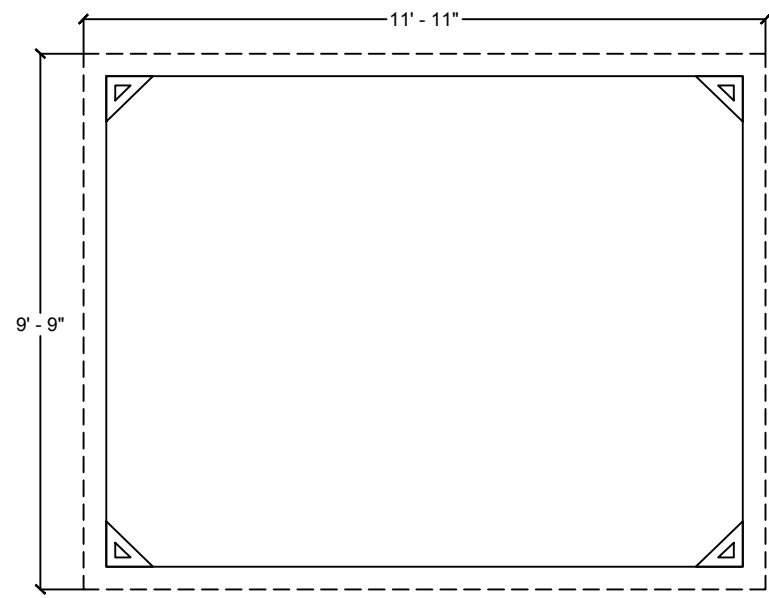
REBORD DU TOIT ROOF OVERHANG
