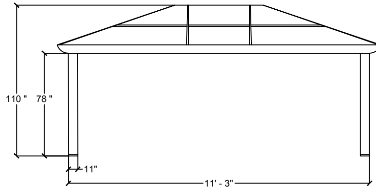
VUE DE CÔTÉ (LONGUEUR) SIDE VIEW (LENGTH)
