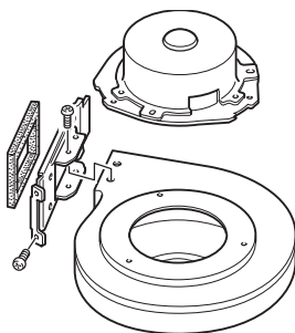
Fan Assembly / Motor
