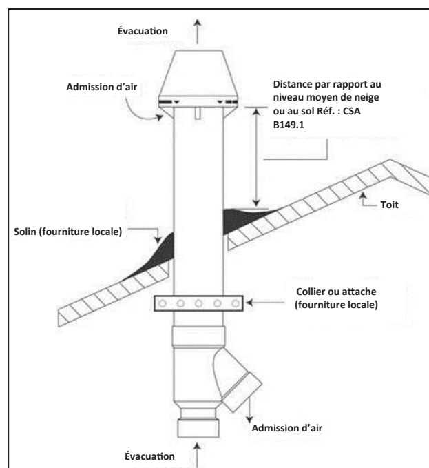
Terminaison par le toit
