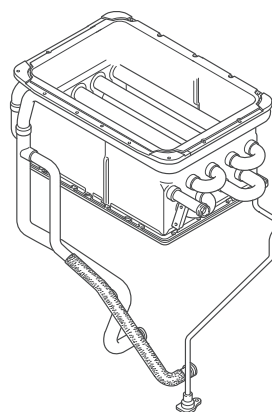
Échangeur thermique
