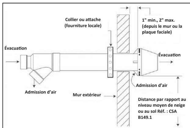
Terminaison dans un mur
