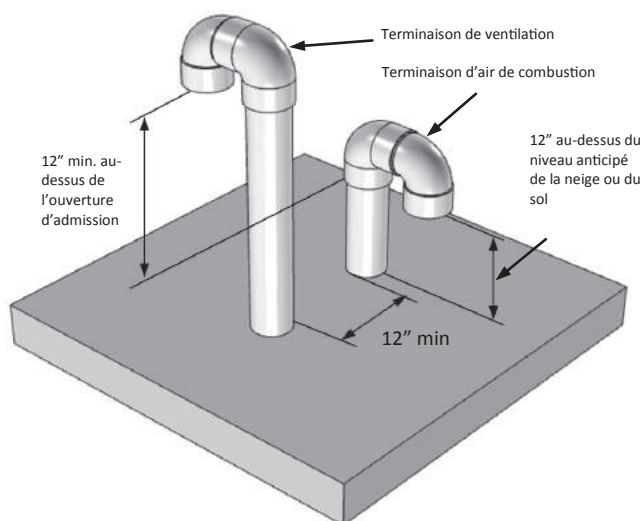
Terminaison verticale de ventilation avec U renversé et tuyau d'air de combustion
