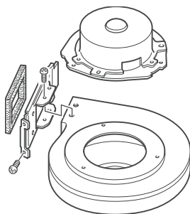
Ensemble de ventilateur/moteur
