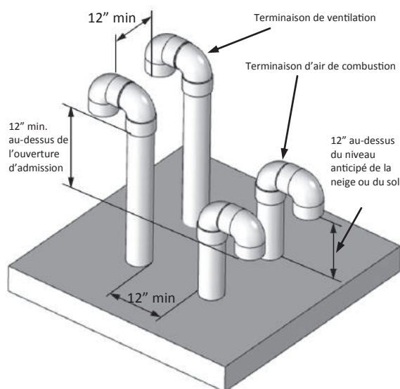
Terminaison verticale de plusieurs chauffe-eau
