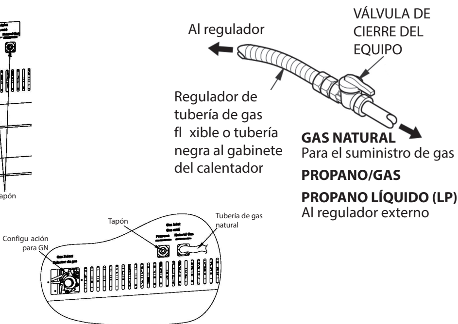
Fig. 16—Conexión de la línea de gas flexible
