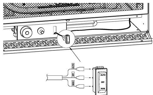
Fig. 9—Conexión del interruptor
