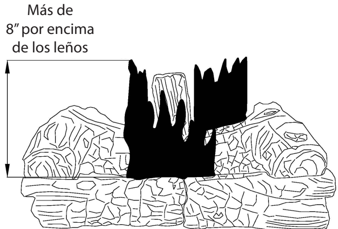
Fig. 25: Patrón de llama incorrecto del quemador
