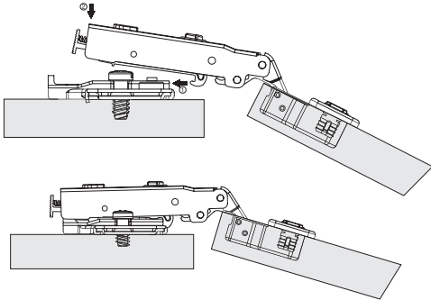
105° Hinge
