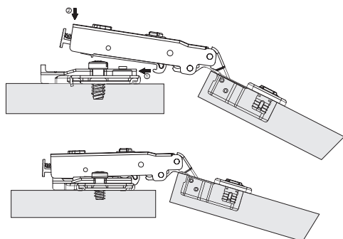
Bisagra de 105°
