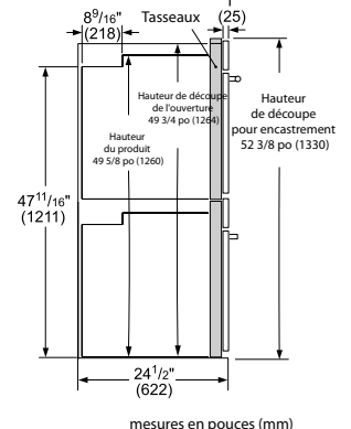
Vue latérale
