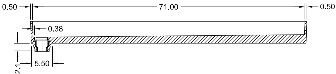
SECTION A-A
