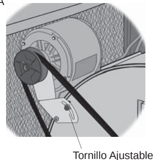
Tornillo Ajustable
