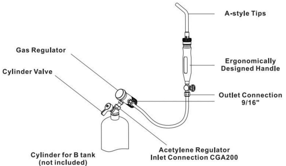
Brenneraufbau
