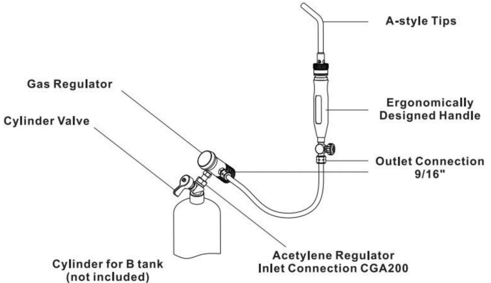
Fakkelopstelling
