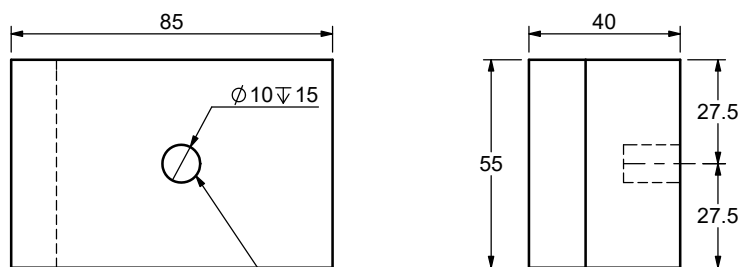
Insert nut M8x15
