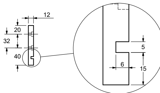
DETAIL AO SCALE 1 : 1
