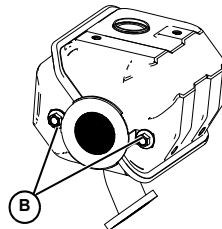
Imagen 4-12. Fijaciones del supresor de chispas
