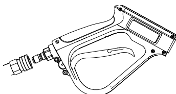
Figure 2-15. Raccordement du tuyau à haute pression au pistolet pulvérisateur - Raccord rapide
