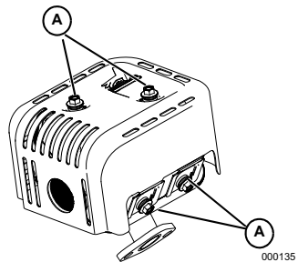
Figure 4-11. Attaches de la protection thermique
