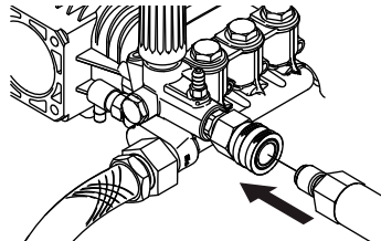
Imagen 2-13. Conexión de la manguera de alta presión a la bomba triple
