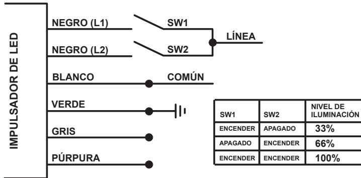
CABLEADO DE LEDS DE 120-277 VOLTIOS
