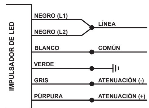
CABLEADO DE LEDS DE 120-277 VOLTIOS
