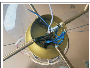
Step 3. Install luminaire
