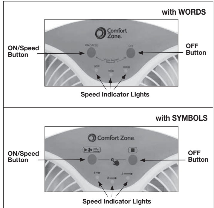
Fig. 8 FAN SPEED CONTROL PANEL
