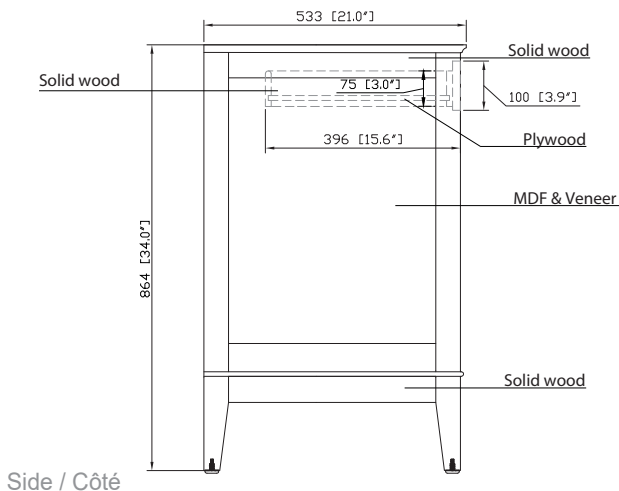
Side / Côté
