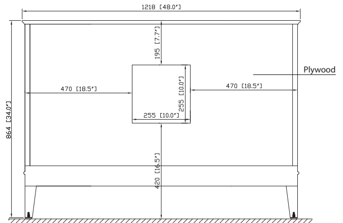
Back / Derrière
