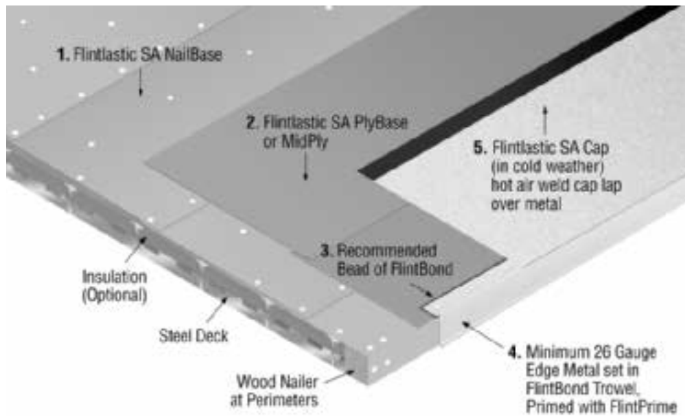
Edge Detail 3 Ply
