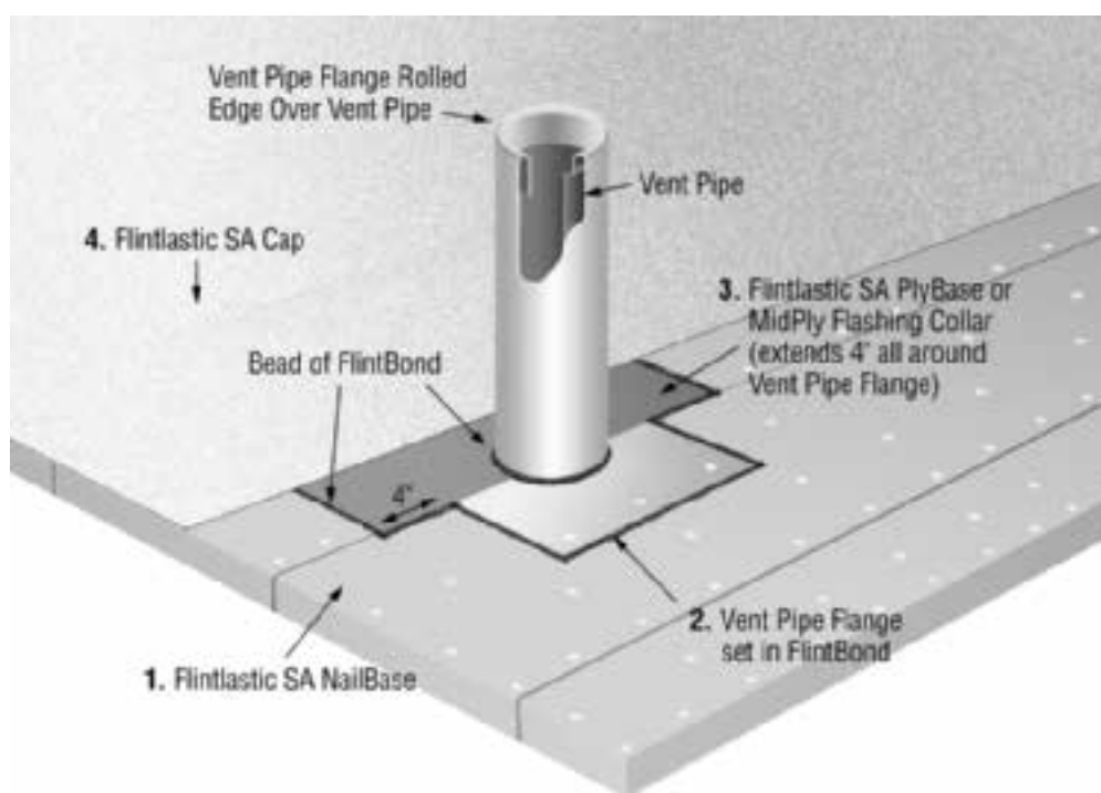
Vent 2 Ply
