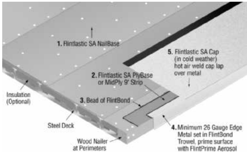
Edge Detail 2 Ply
