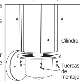
Figura 10 Unidades cilíndricas
