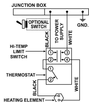
C-2 STANDARD SINGLE ELEMENT 120 VOLT & 277 VOLT
