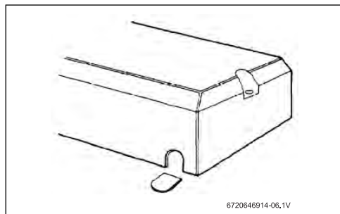
Fig. 9 Découpe de la languette du capot
