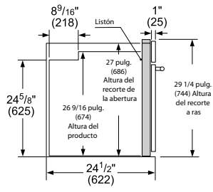
Vista lateral
