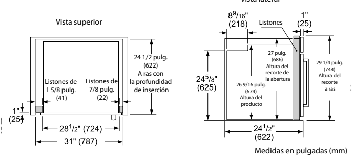
Instalación a ras
