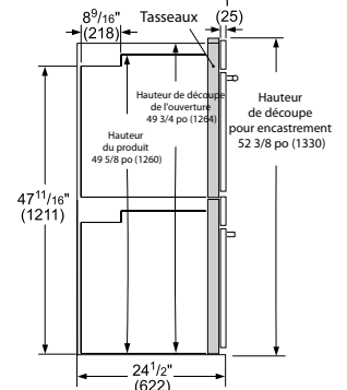
Vue latérale
